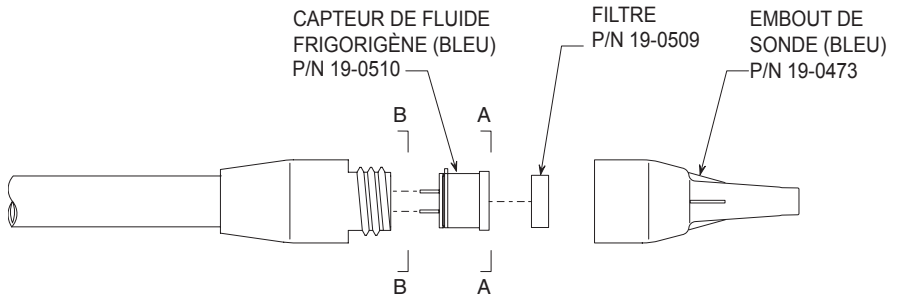
CAPTEUR DE FLUIDE FRIGORIGÈNE
