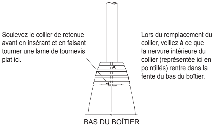
Figure 6. Installation du collier de retenue avant
