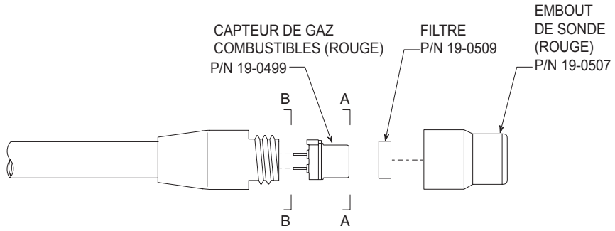
CAPTEUR DE GAZ COMBUSTIBLES
